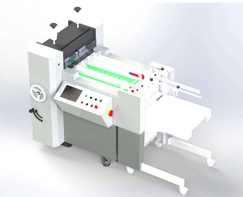
rotatie stansmachine
